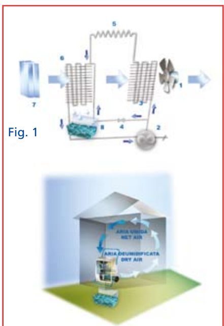
1. Ventilatore - 2. Compressore - 3. Condensatore - 4. Valvola by-pass (Fig. 1) - 5. Tubo capillare (Fig. 1) - 6. Evaporatore - 7. Filtro aria - 8. Vaschetta raccolta acqua - 9. Umidostato - 10. Spia vaschetta piena - 11. Spia di sicurezza - 12. Interruttore - 13. Contatore
